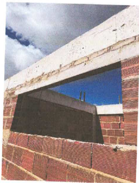
Fixação (encunhamento) de alvenaria de vedação com tijolo maciço
