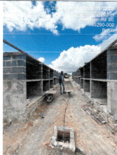
ALVANRIA E LAJE DAS GAVETAS, E CAIXA DE PASSAGEM E ELETRODUTOS
