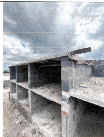
FORMA DAS LAJES DAS GAVETAS
