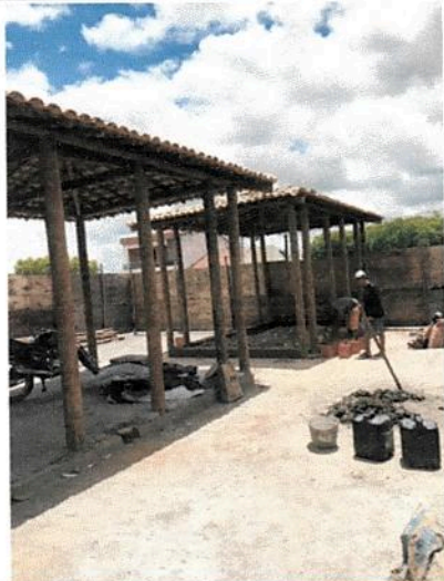
Estrutura do telhado mais início do piso
