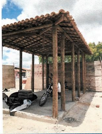
Estrutura do telhado
