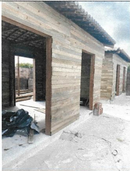
Estrutura em madeira das paredes
