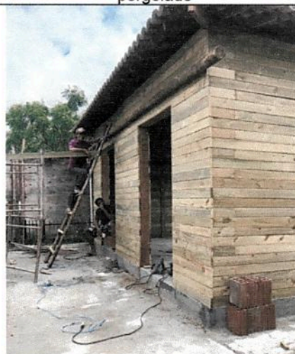
Estrutura em madeira das paredes e início da estrutura do pergolado
