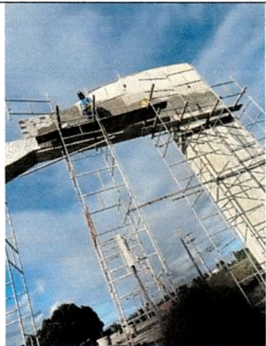
Volumes e acabamentos de viga – Via Tomar do Geru
