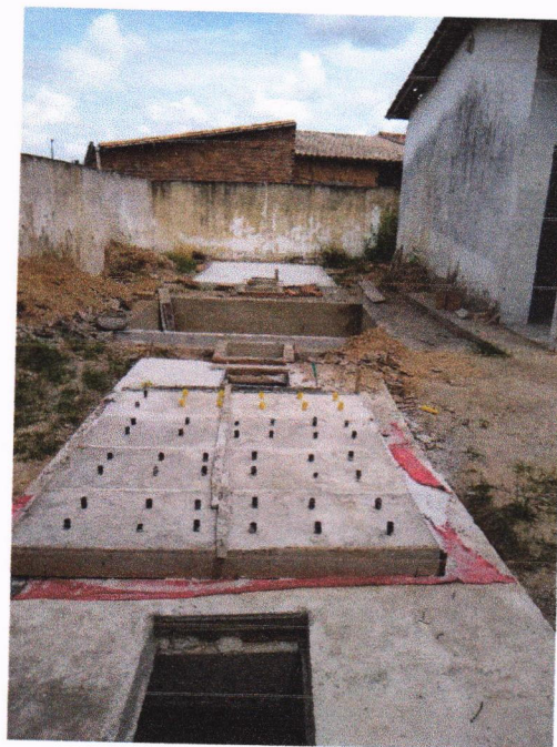
Unidade de tratamento de esgoto
