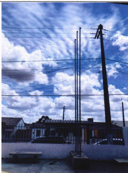
Mastro com 3 tubos de aço galvanizado
